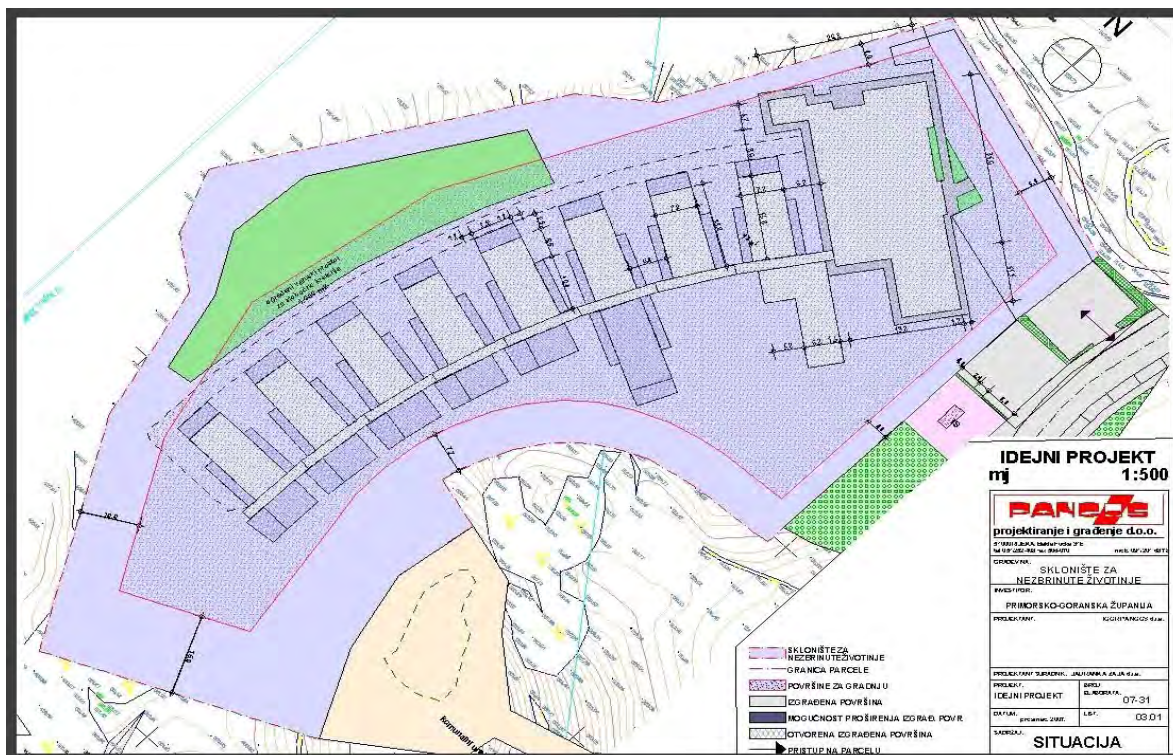
slika 4.: Sklonišče za napuštene živali - situacija
